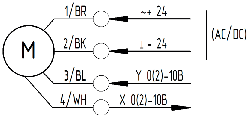
Схема подключения аналоговых приводов с обратной связью.
